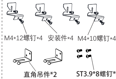
1645073 集成顶用安装配件包*1
